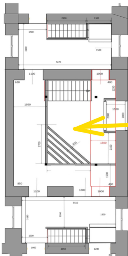
План 1 этажа
